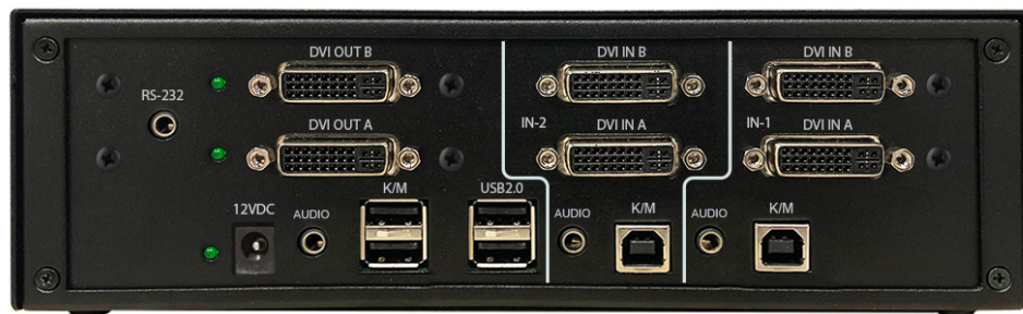
SM-DVN-2D Back
